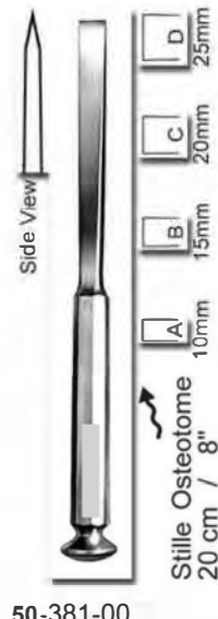
50-381-00 Stille Osteotome 20 cm / 8"
